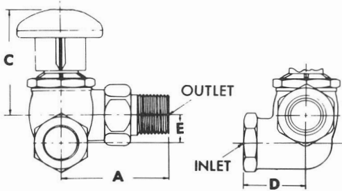
FIG. 7 MODEL RH1
